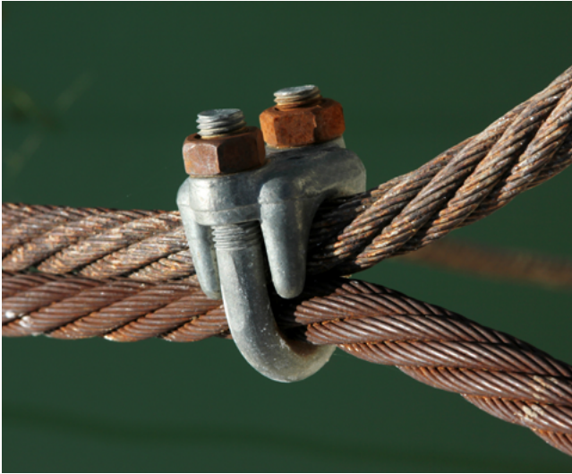
Figura 26. Cable deteriorado
